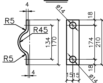
Развертка поз.5
